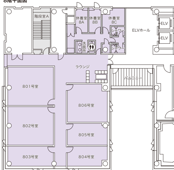
8階平面図
