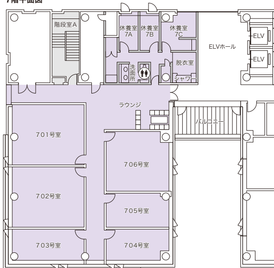
7階平面図
