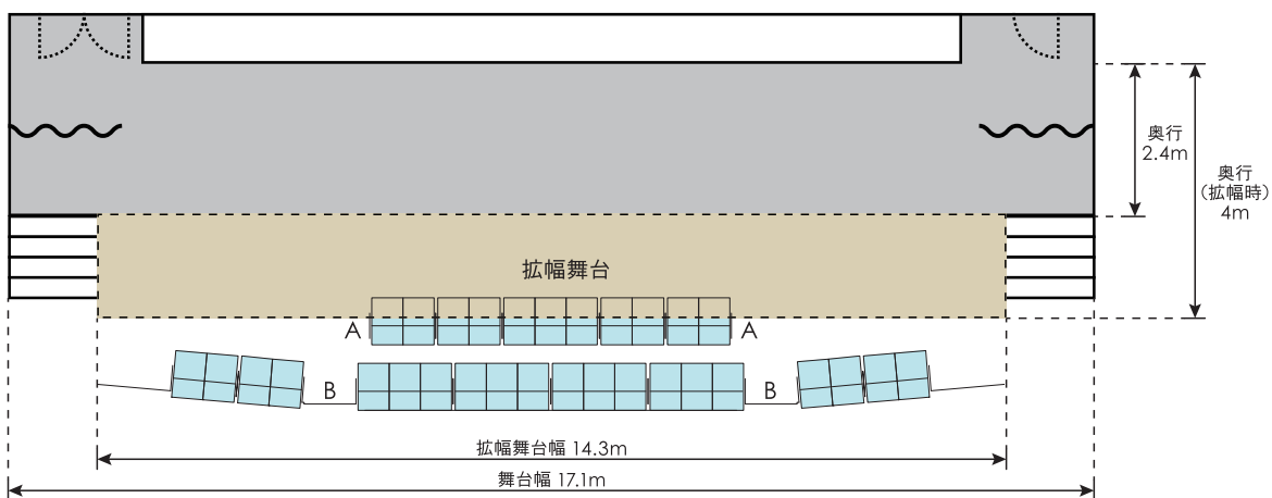
舞台平面図
