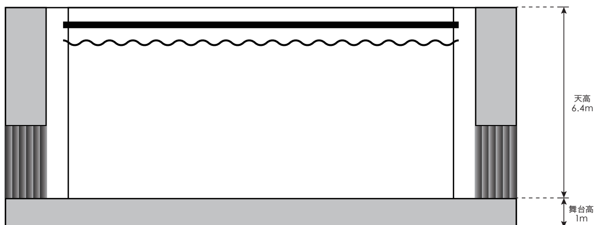
舞台正面図
