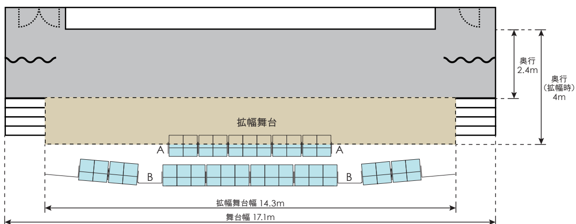
舞台平面図
