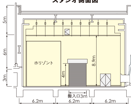
スタジオ側面図
